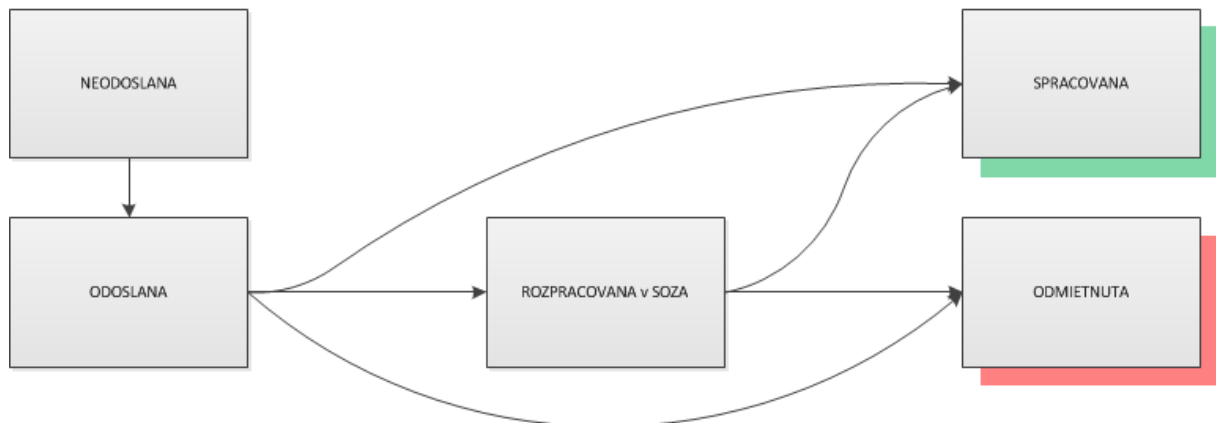
Obrázok 11: Stavy nahlášky v ISpA
